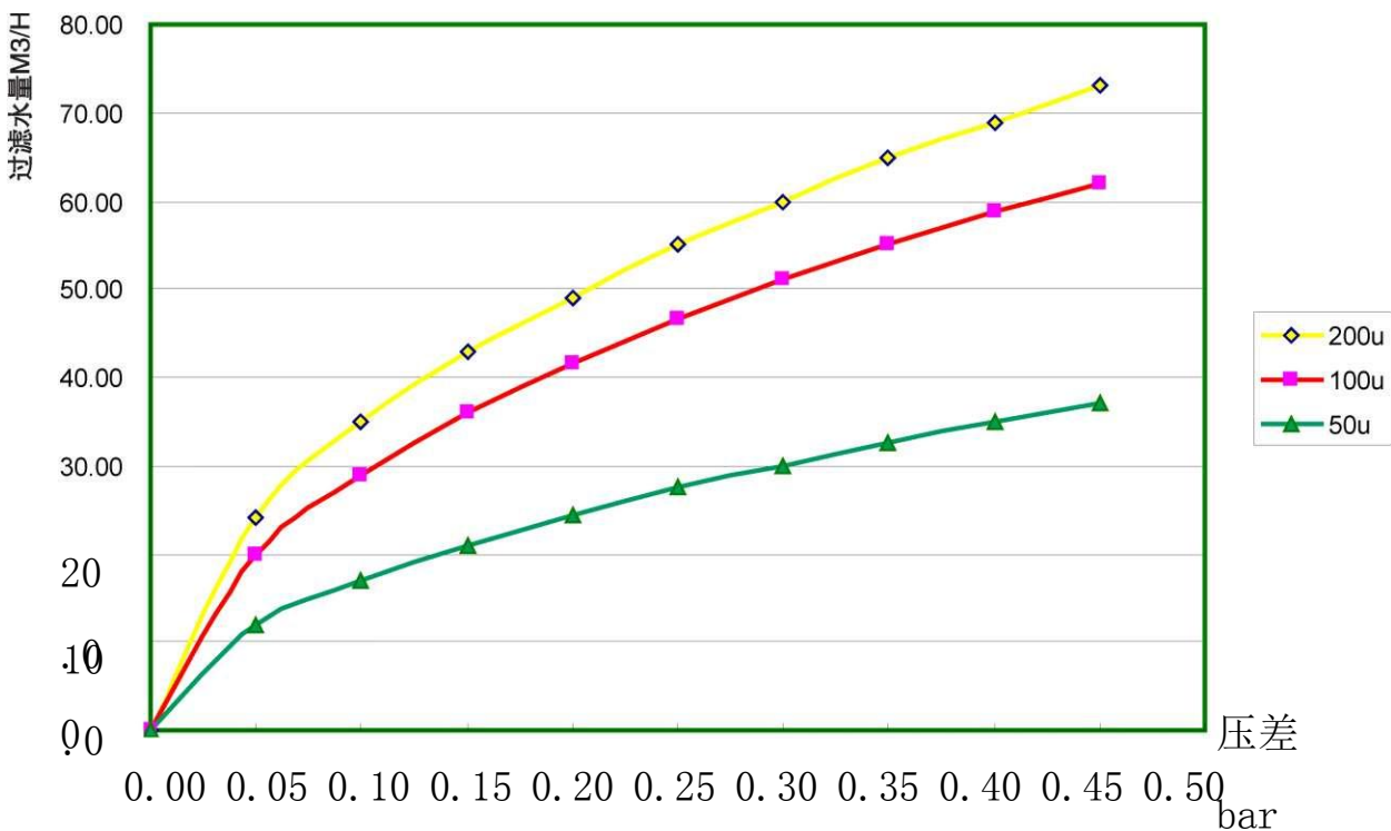
RLZD3 过滤单元流量 Vs 压差曲线
